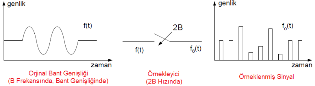
Şekil 2.1: Örnekleme teoremi
