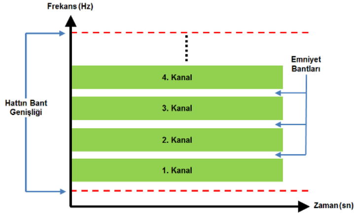
Şekil 1.11: Frekans bölmeli çoklama (FDM)
