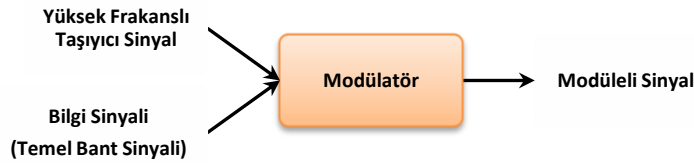
Şekil 1.3: Genlik modülasyonu blok şeması
