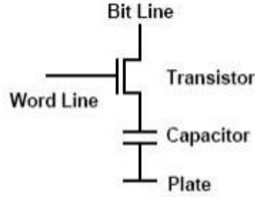
Şekil 1.3: DRAM bellek hücresi
