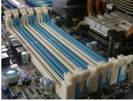
Resim 2.7: DIMM RAM slotu
