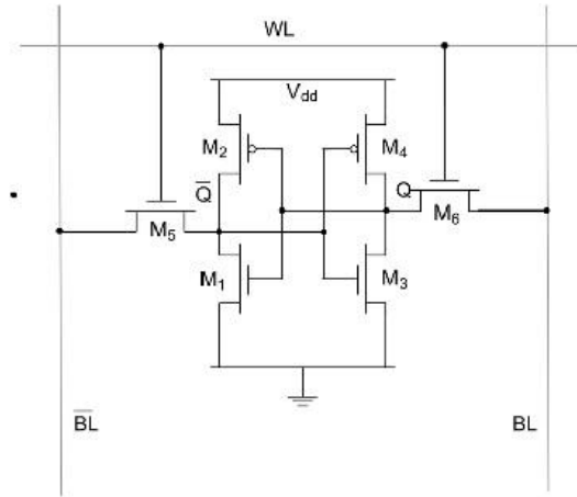
Şekil 1.2: SRAM bellek hücresi
