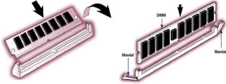
Şekil 2.1: 72 pin SIMM ve 168 pin DIMM takılması
