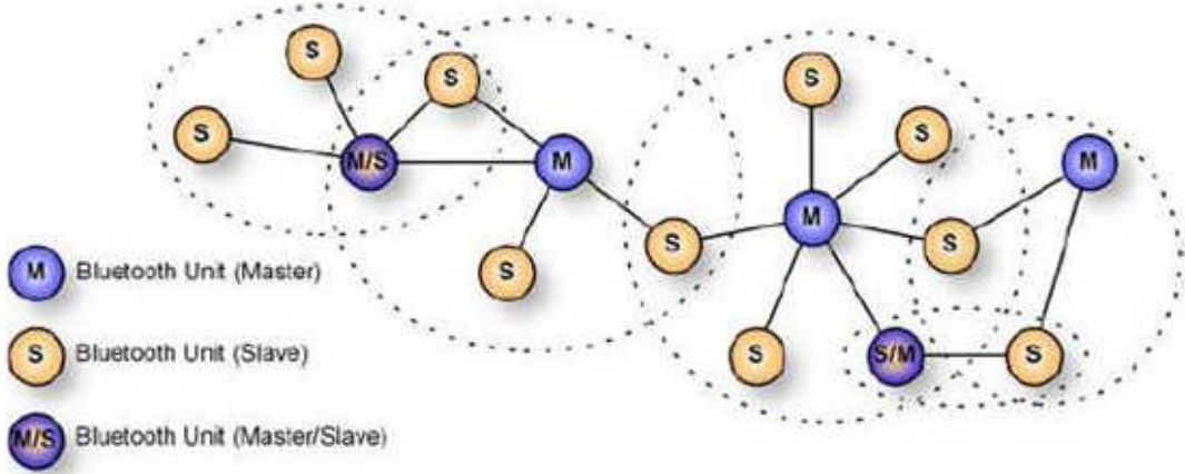
Şekil 2.2: Scatternet topolojisi şematik gösterimi
