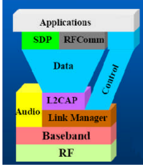
Resim 2.15: Bluetooth teknolojisi protokol kümesi
