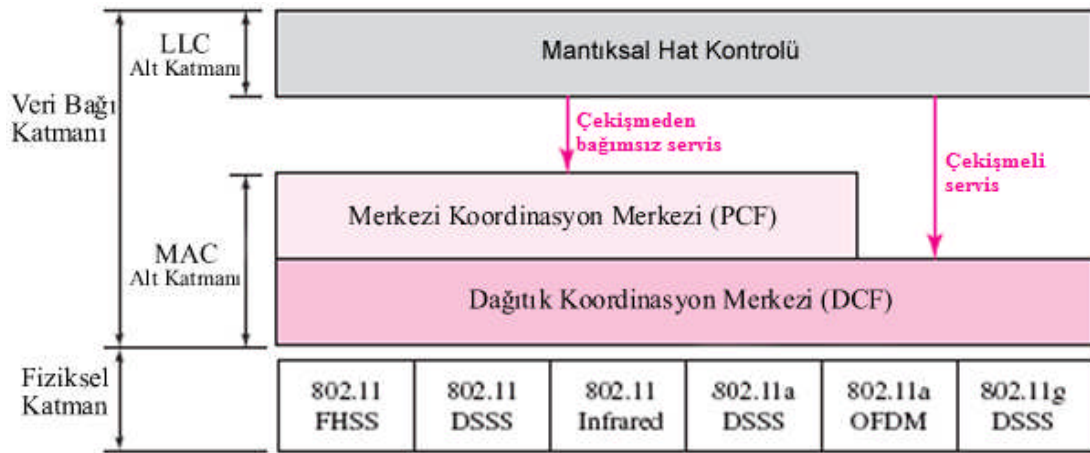
Resim 1.16: OSI başyuru modeli MAC alt katmanı
